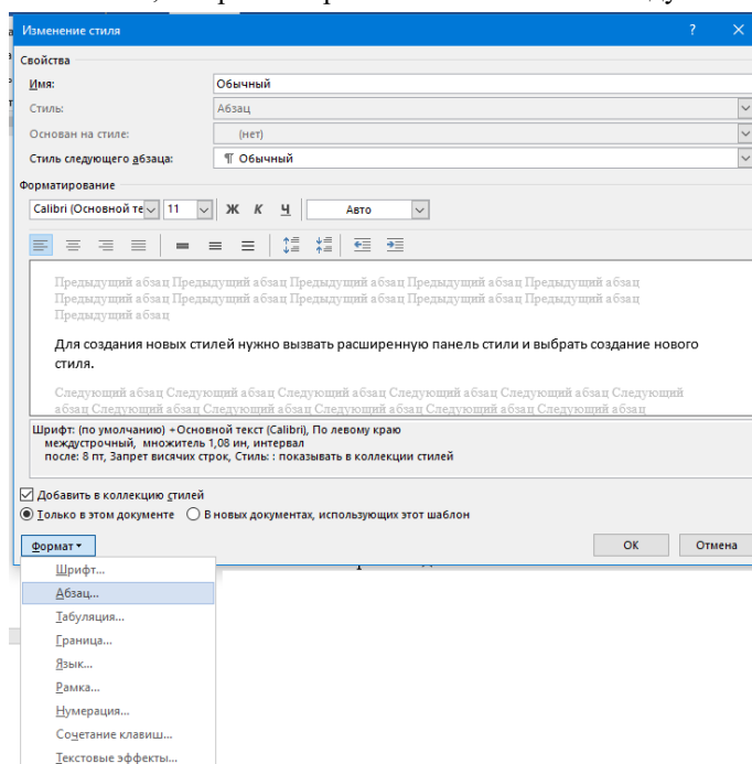
Рисунок 2 - Изменение стиля
