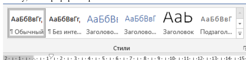
Рисунок 1 - Стили
