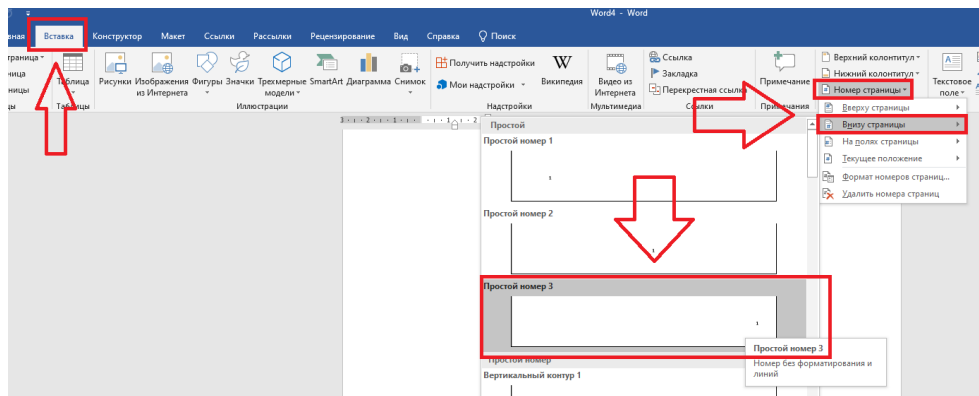
Рисунок 5 - Нумерация страниц
