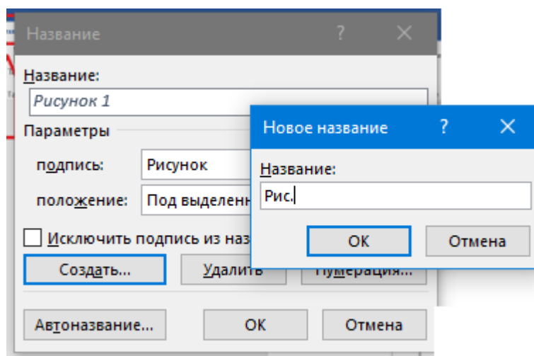
Рисунок 6 - Наименование рисунков
