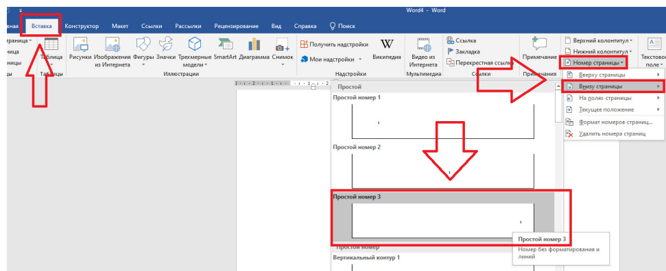
Рисунок 5 - Нумерация страниц
